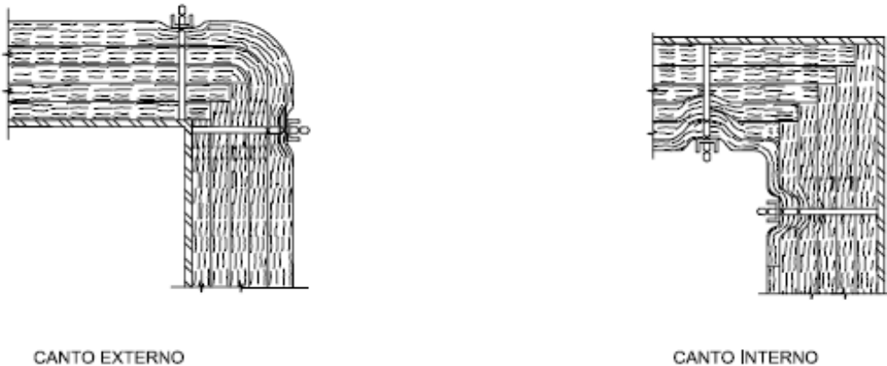
Figura 02 e 03: Detalhe da montagem nos cantos.
