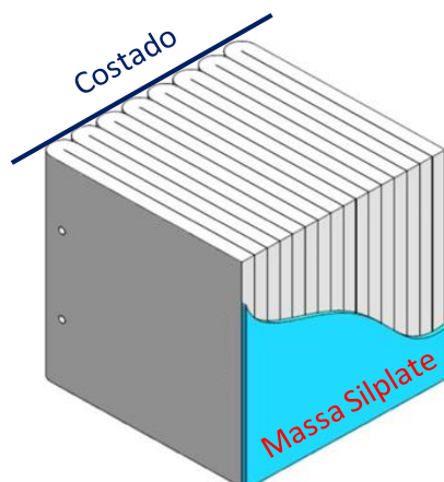
Layot de direcionamento para instalação dos módulos
