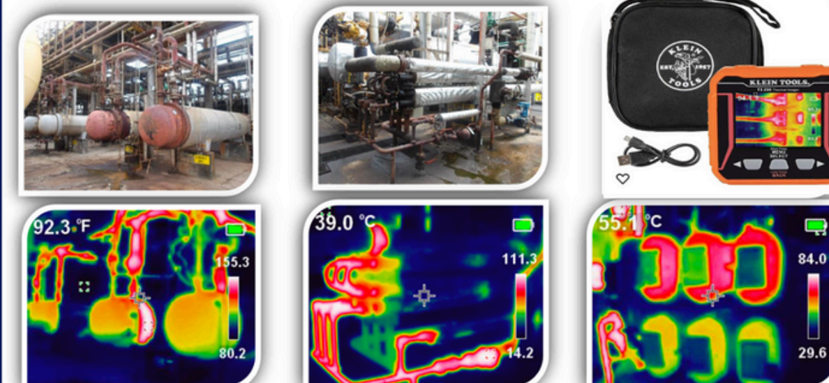
AVALIAÇÃO TERMOGRÁFICA
