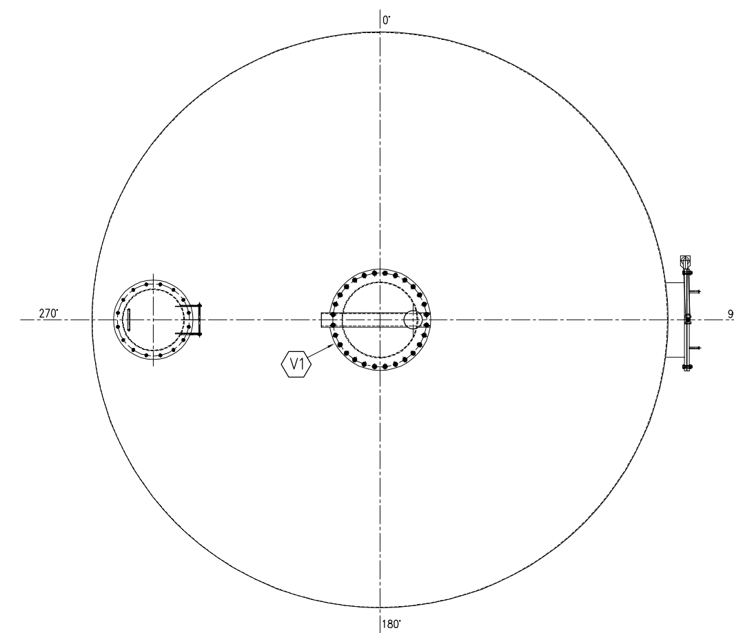
PLANTA - ORIENTAÇÃO DOS BOCAIS PLAN - NOZZLES ORIENTATION HOLD
